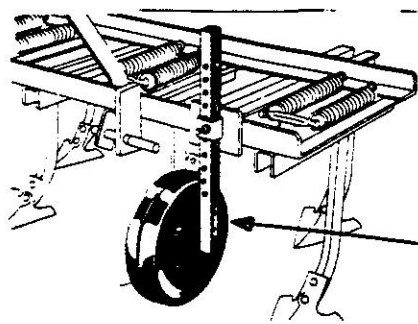
Ruotino regolazione profondità Depth adjusting wheels Petites roues de réglage à pro- fondeur
